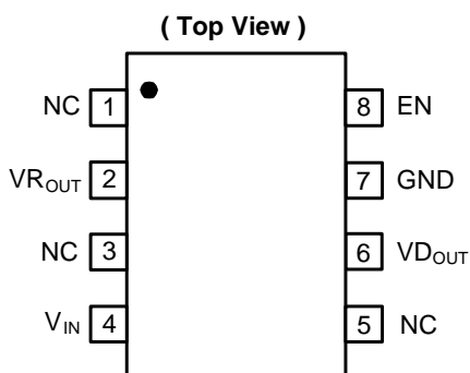
(1) SOP-8L
