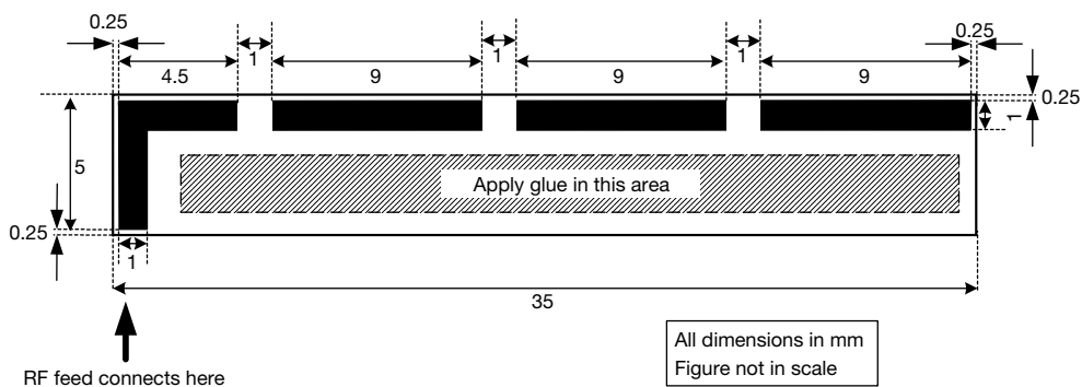
Fig. 5 - VJ 3505 Footprint
