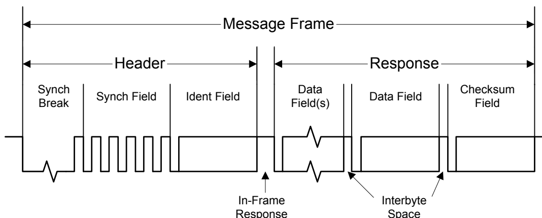
Figure 14-4. LIN Message
