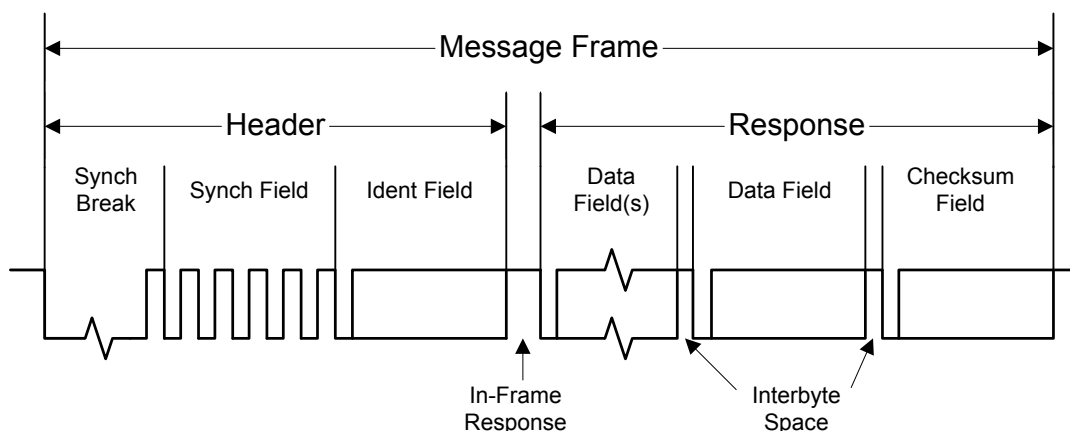
Figure 13-4. LIN Message
