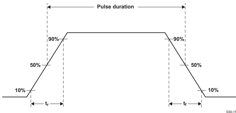
Figure 6-62. UART IrDA Pulse Parameters
