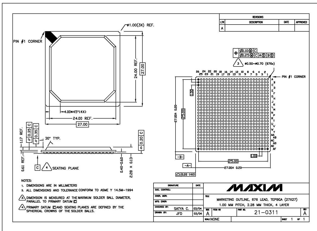
Figure 15-1. 676-Ball TEPBGA
