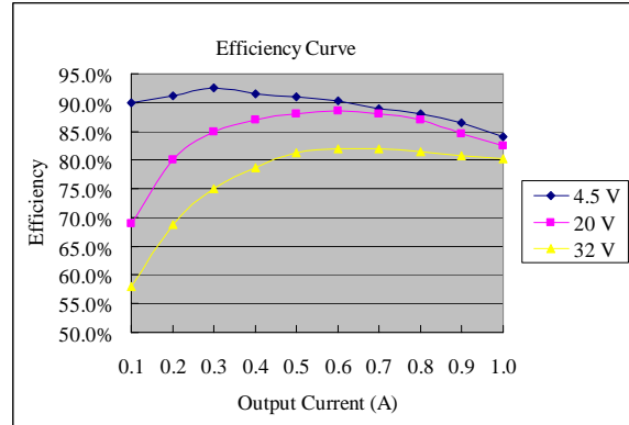
Vo = 2.5 V
