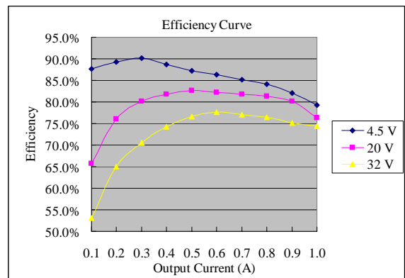
Vo = 1.5 V
