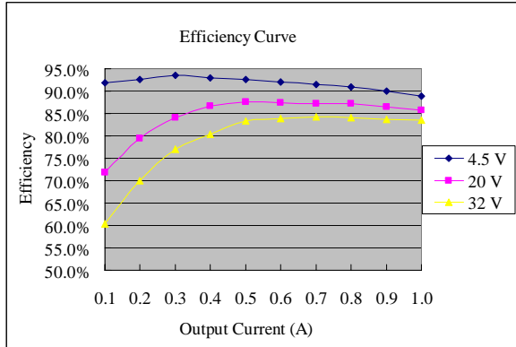
Vo = 3.3 V
