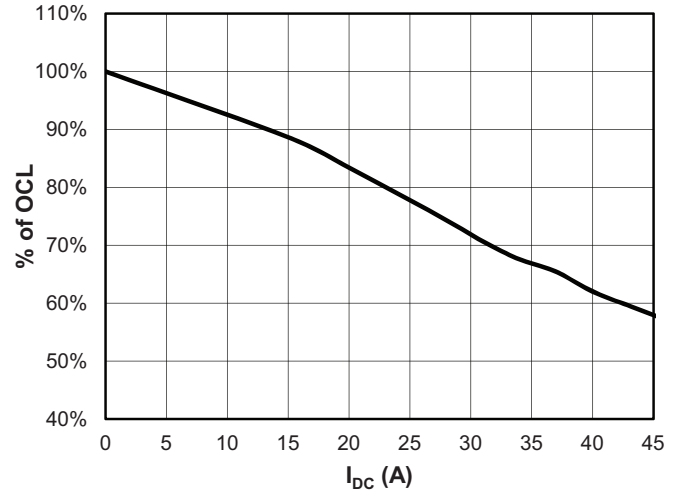
HCM0703-R68-R
