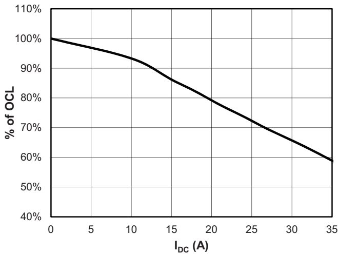
HCM0703-1R5-R
