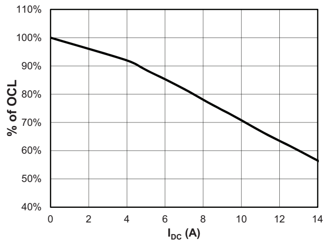
HCM0703-150-R
