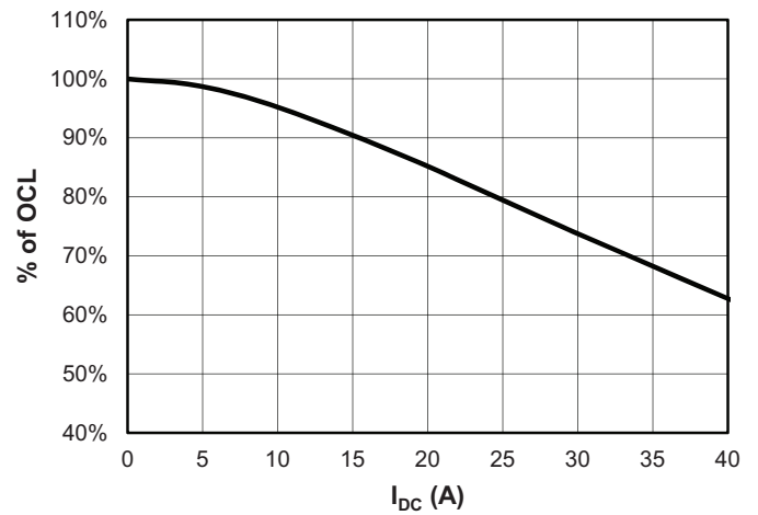
HCM0703-1R0-R
