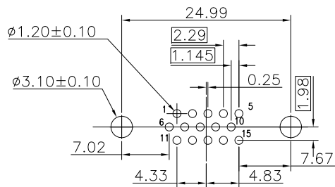
P.C.B LAYOUT(FOR 15P)
