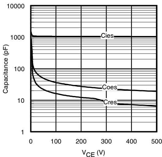
Fig. 17 - Typ. Capacitance vs. V_{CE}
