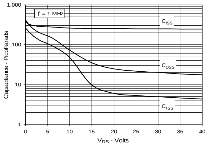
Fig. 11. Capacitance
