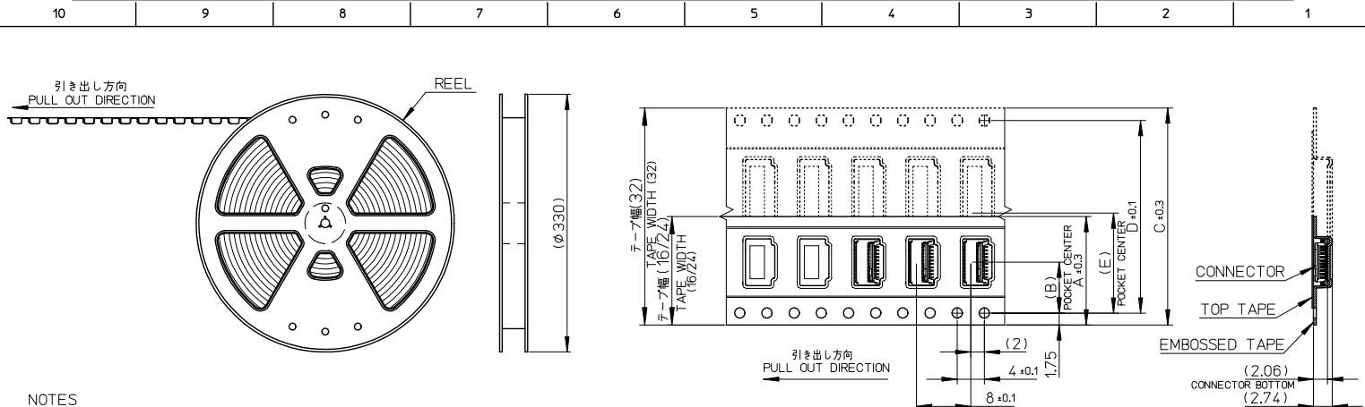
エンボステープ内の製品の向き DIRECTION OF CONNECTOR IN EMBOSSED TAPE
