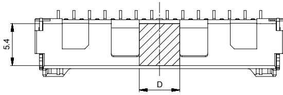
吸着エリア 6~15極 VACUME AREA 6~15CKT
