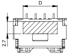
吸着エリア 2~4極 VACUME AREA 2~4CKT
