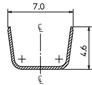
SEC' : D-D*
