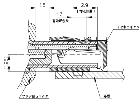
コネクタ嵌合図 (SCALE 8:1)
