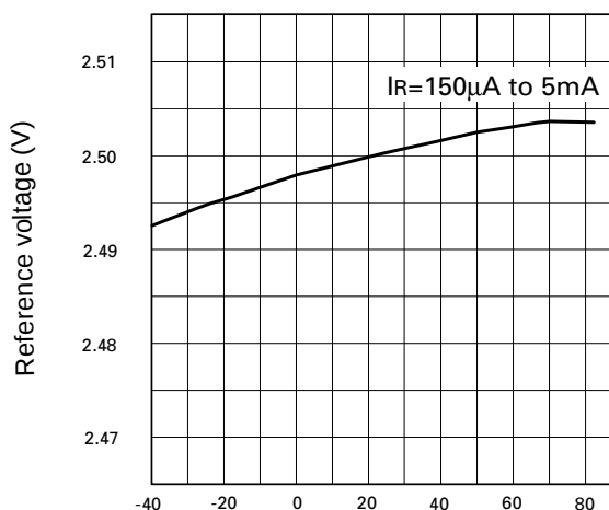
Temperature (°C) Temperature Drift
