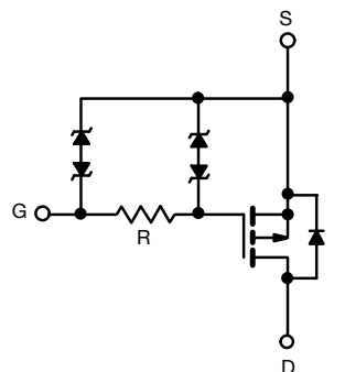
P-Channel MOSFET
