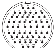
36A66 52 #16(A-c,h-AK) 4 #12(d,e,f,g)
