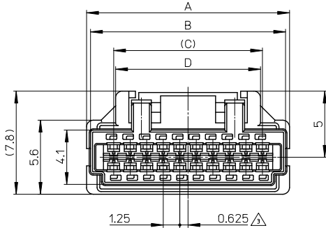
ターミナル装着図 TERMINAL ASSEMBLY DRAWING
