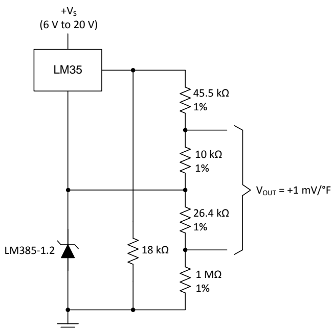
Figure 21. Fahrenheit Thermometer
