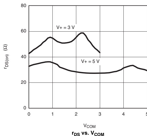
r_{DS} vs. V_{COM}
