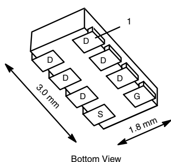
1206-8 ChipFET®
