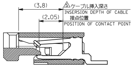
断面D-D SECT.D-D
