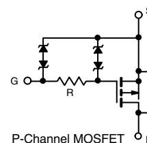
P-Channel MOSFET
