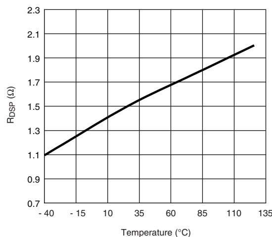
DH R_{DSP} vs. Temperature
