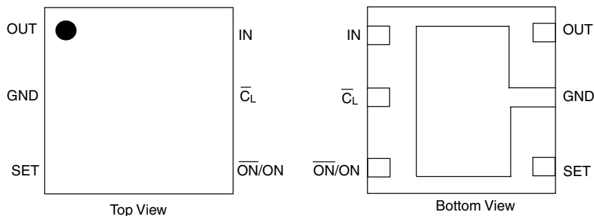
TSC75-6 PACKAGE
