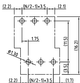
P.C.B LAYOUT
