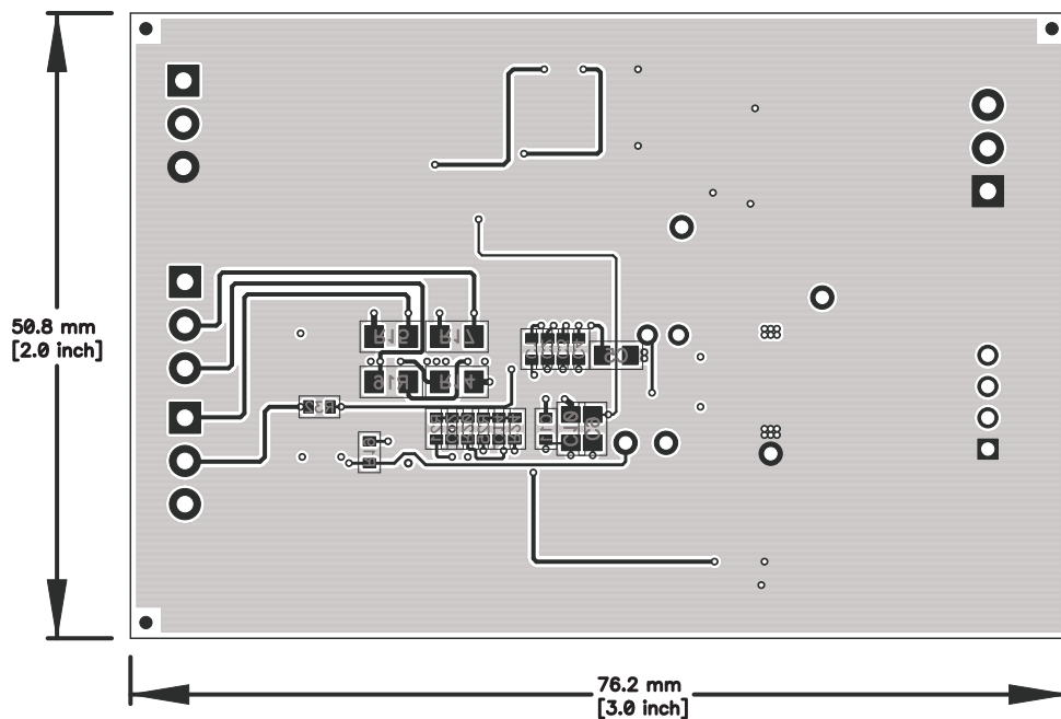
Figure 24. Bottom Layer
