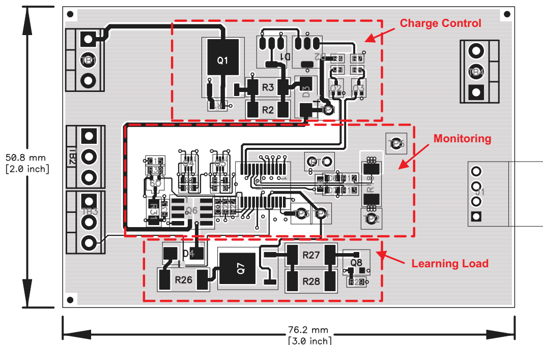
Figure 21. Top Layer
