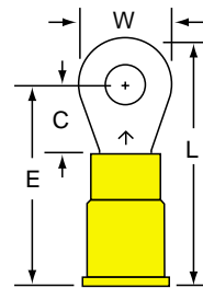
MV10-8R Stud Size 8 Wire Range 12-10
