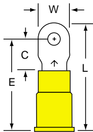
MV10-4R/S Stud Size 4 Wire Range 12-10
