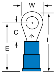
MV14-10R Stud Size: 10 Wire Range: 16-14
