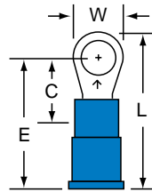
MV14-8R/S Stud Size: 8 Wire Range: 16-14
