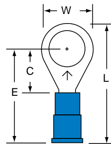
MV14-516R/S Stud Size: 5/16 Wire Range: 16-14
