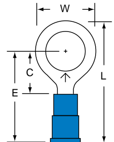
MV14-38R Stud Size: 3/8 Wire Range: 16-14
