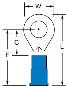
MV14-14R/S Stud Size: 1/4 Wire Range: 16-14
