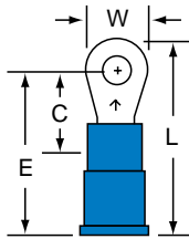
MV14-4R/S Stud Size: 4 Wire Range: 16-14
