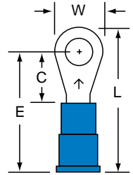
MV14-8R/L Stud Size: 8 Wire Range: 16-14
