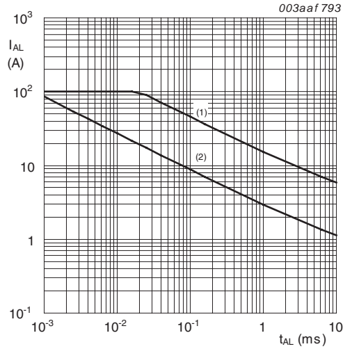
(1) T_{j(jrrt)} = 25^\circ C ; (2) T_{j(jrrt)} = 100^\circ C
