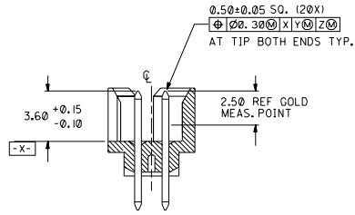
SECTION G-G SCALE - 4 : 1
