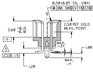
SECTION G-G SCALE - 4 : 1
