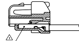
ターミナル装着図 TERMINAL ASSEMBLY DRAWING
