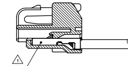
ターミナル装着図 TERMINAL ASSEMBLY DRAWING
