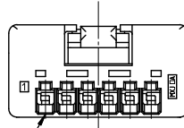
回路番号 1 CKT NO. 1
