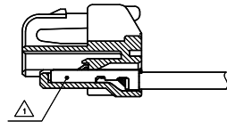
ターミナル装着図 TERMINAL ASSEMBLY DRAWING
