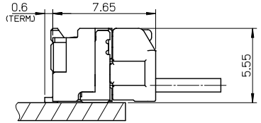
嵌合図
