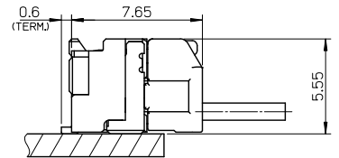
嵌合図
