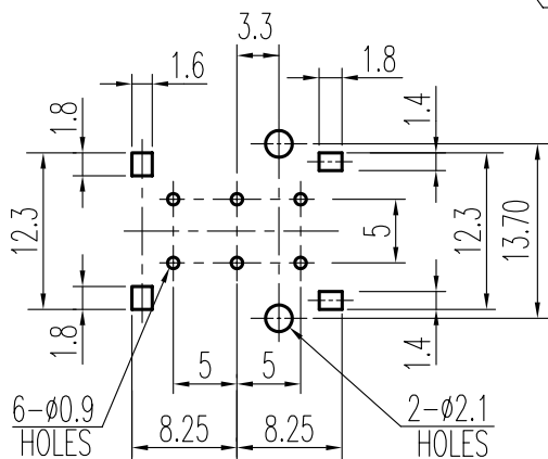
安装孔 PIERCING PLAN
