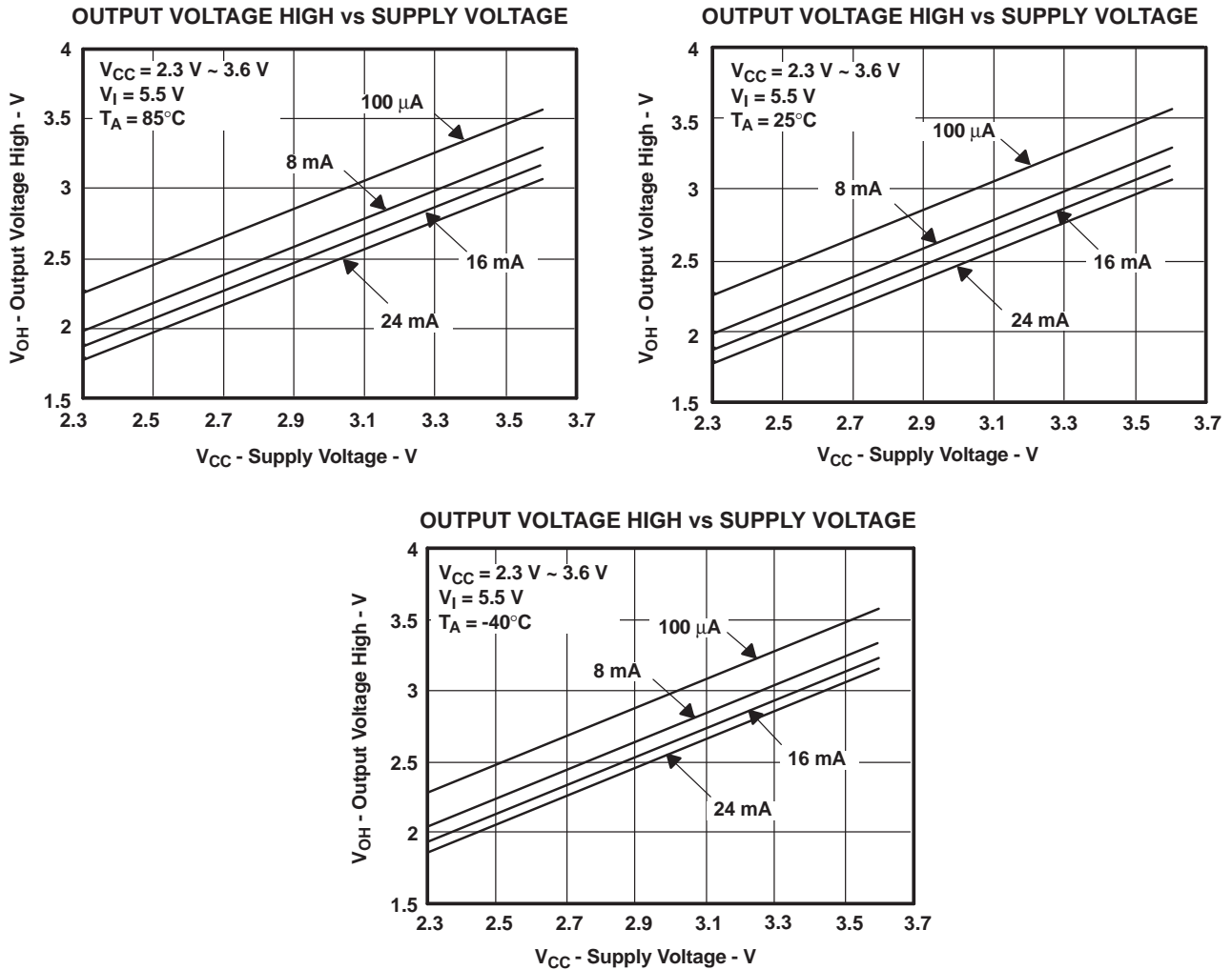
Figure 4. V_{OH} Values
