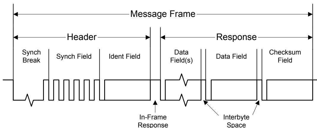
Figure 12-4. LIN Message
