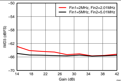
Figure 45. IMD3
