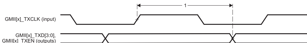
Figure 7-9. GMII[x]_TXD[3:0], GMII[x]_TXEN Timing - MII Mode
