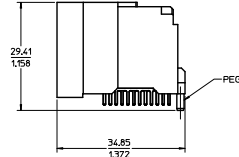
75556-15** SHOWN (W/PEG)
