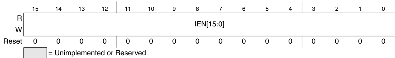
Figure 16-12. ATD Input Enable Register (ATDDIEN)
