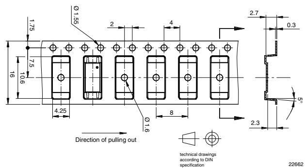
Fig. 21 - Tape Dimensions
