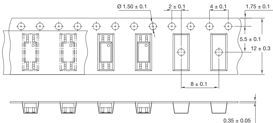
Fig. 19 - Tape Dimensions
