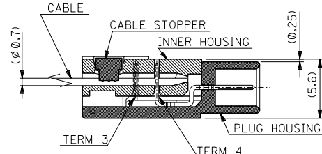
SECT C-C (SCALE:4-1)
