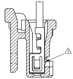
ターミナル装着図 TERMINAL ASSEMBLY DRAWING
