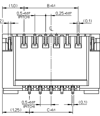
アクチュエータ開放位置 ACTUATOR OPENING POSITION
