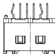
6~7 極形状 (ロック面及び反ロック面)
