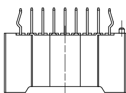
8~10 極形状 (反ロック面)
